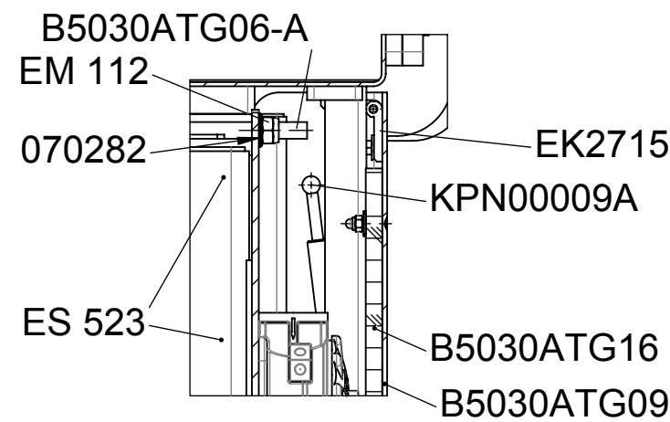
A-A (1 : 5)
