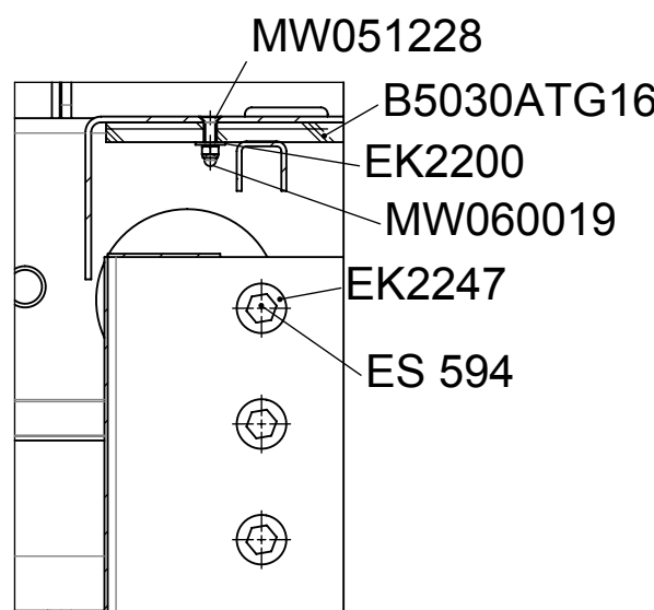
B-B (1 : 5)
